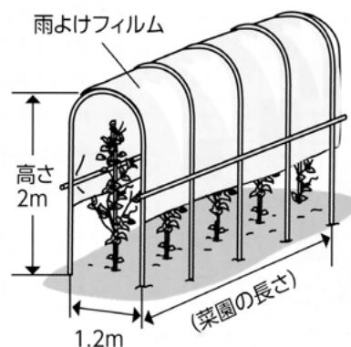
図3 雨よけ
